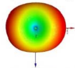
Curved Dipole 1.3 dBi (+z)
